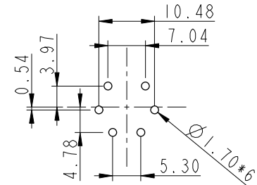
6Pin Male Connector Male Pin PCB Layout 6Pin 公接頭 PCB挖孔位置尺寸圖
